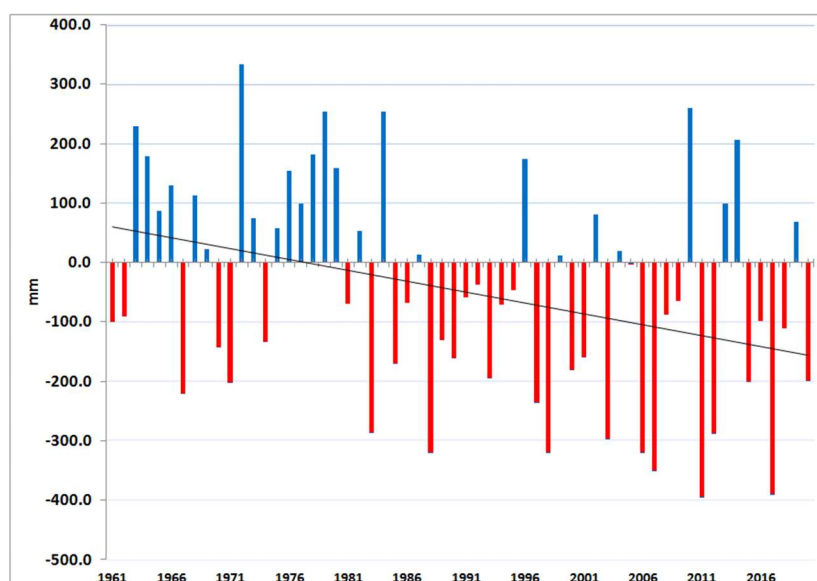
Figura 8 - Serie del valore medio regionale del bilancio idroclimatico annuo (fonte Arpaè)
