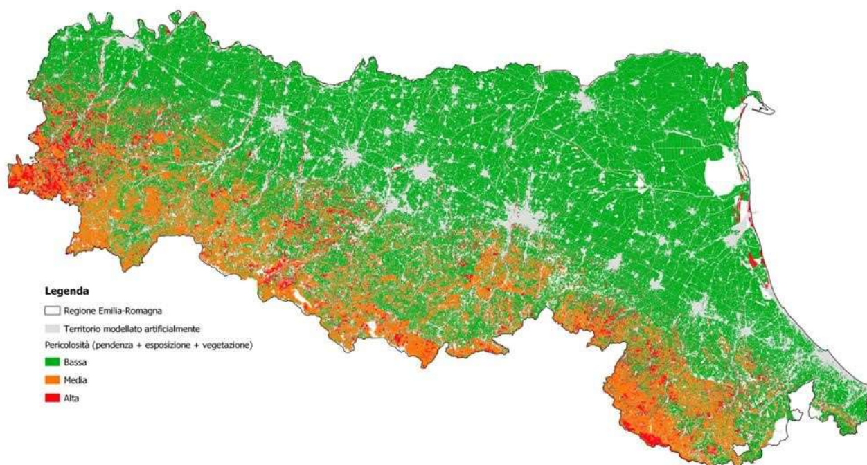
Figura 4: Carta delle aree a pericolosità
